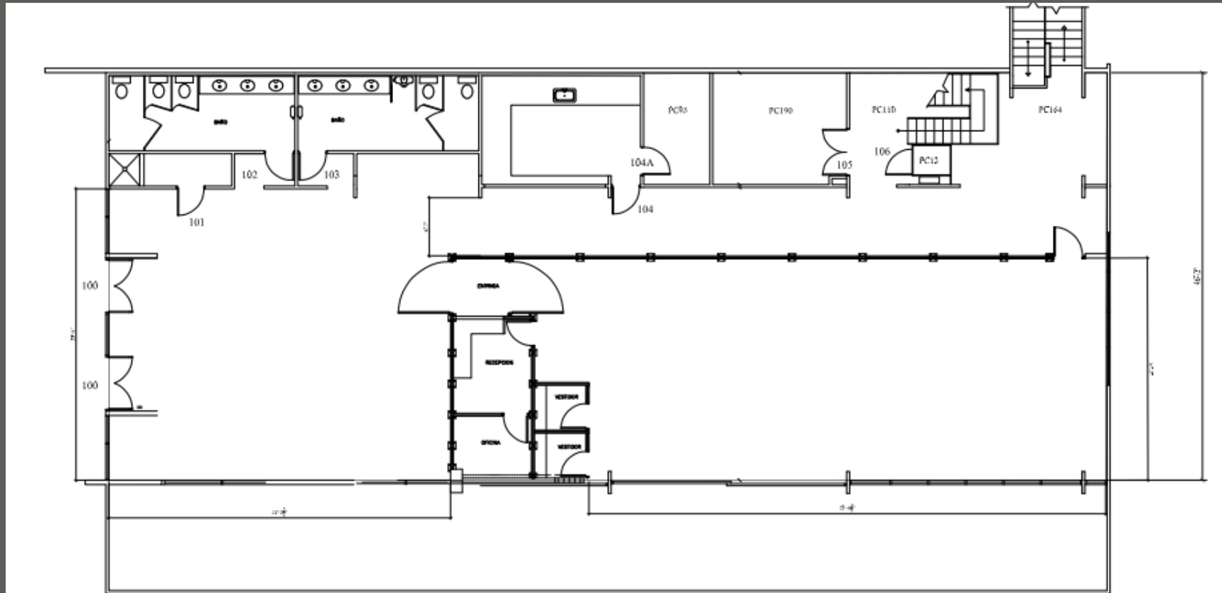
PLANTA DE PISO PRIMER NIVEL PROPUESTO
